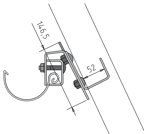
POHLED ZBOKU
