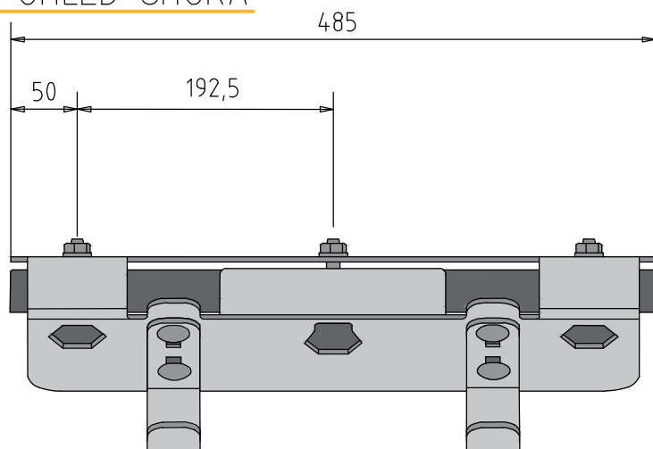
POHLED SHORA
