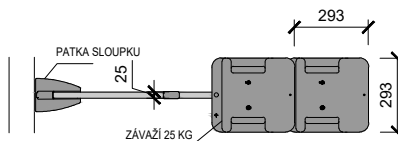
POHLED SHORA
