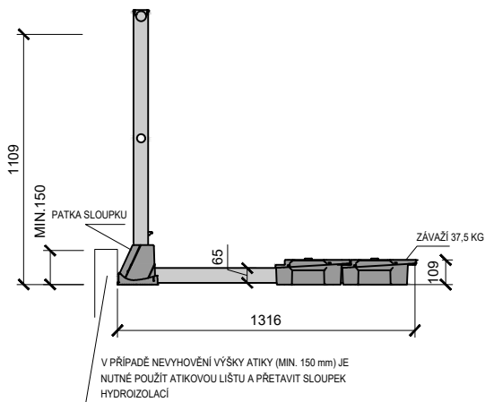
POHLED ZBOKU
