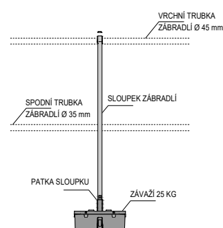
POHLED ZEPŘEDU
