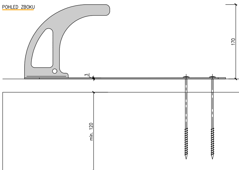
POHLED ZBOKU
