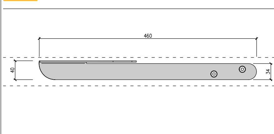
POHLED SHORA
