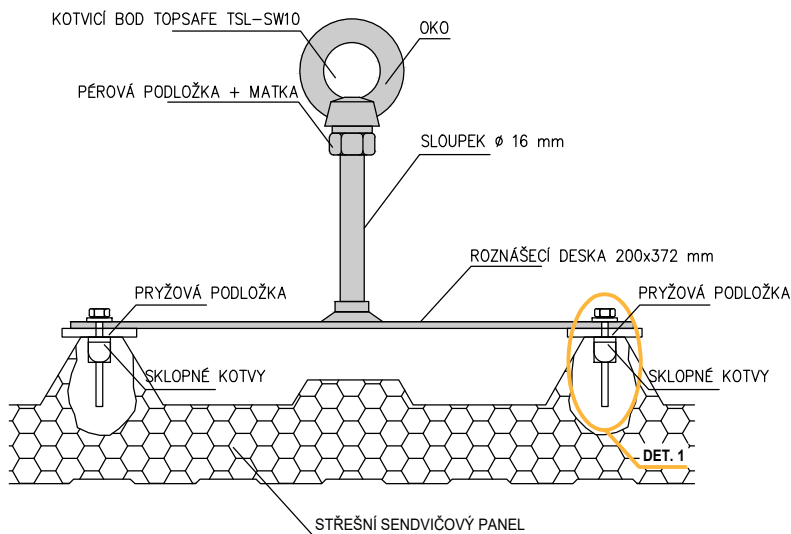
DET. 1 M1:3
